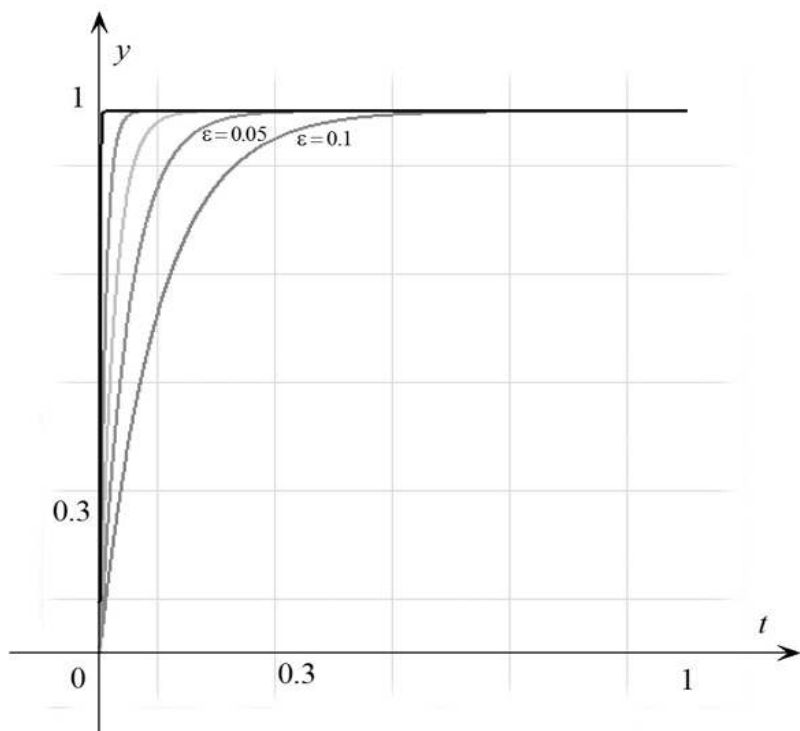
Рис. 5.1. Графики решений краевой задачи для различных \varepsilon > 0
