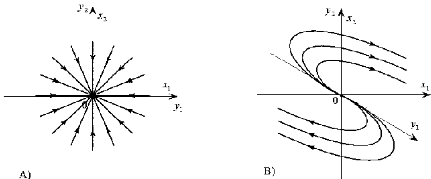
Рис. 6.5. Положения равновесия дикритический узел и вырожденный узел
