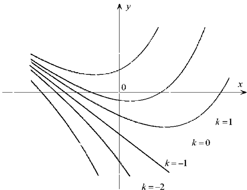
Рис. 1.2. Эскиз семейства интегральных кривых задачи 1.1.1
