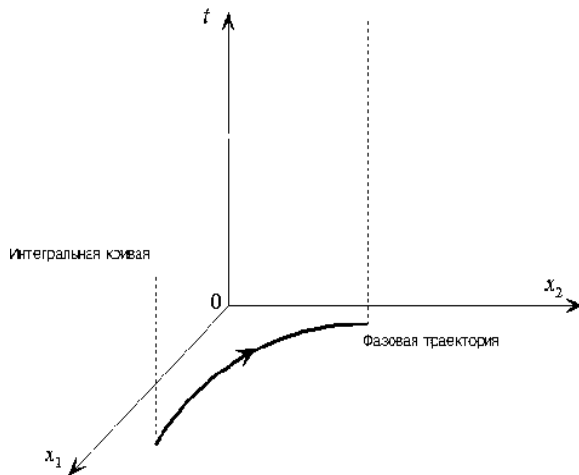
Рис. 6.1. Интегральные кривые и фазовые траектории
