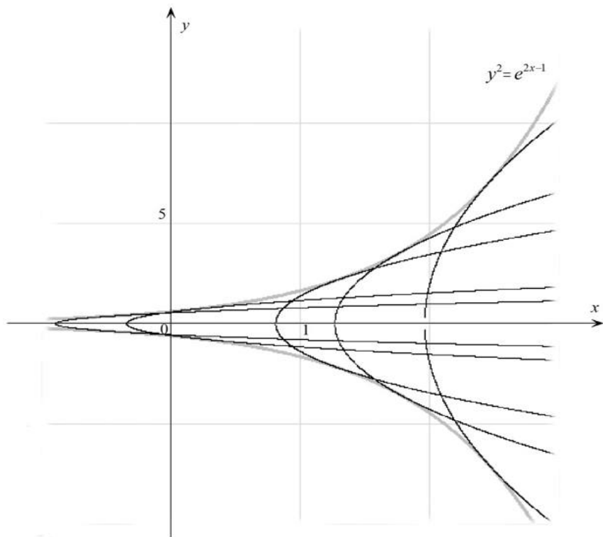
Рис. 1.4. Интегральные кривые для уравнения в задаче 1.5.1
