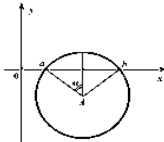
Рис. 7.1. К решению задачи 7.4.2.
