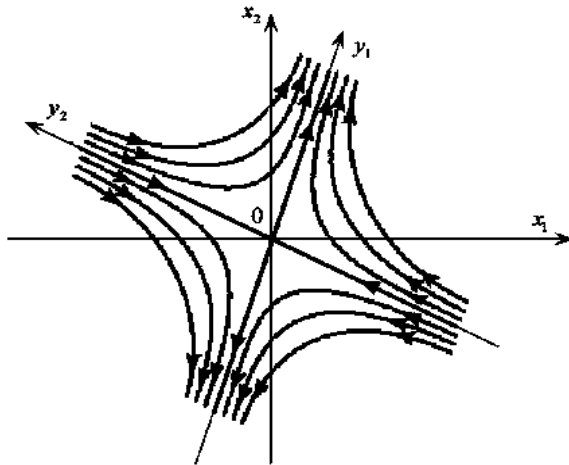
Рис. 6.4. Положение равновесия седло с \lambda_1 > 0, \lambda_2 < 0
